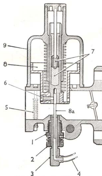
FIG 2:6 A section through SU carburettor
